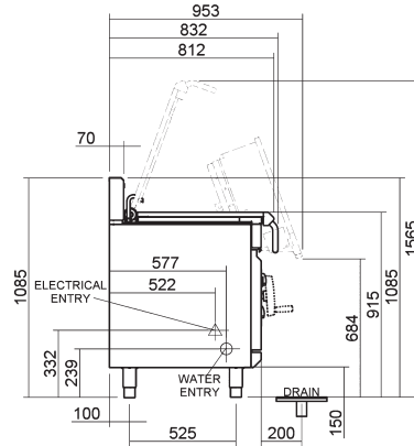
E580-12, E580-12E
