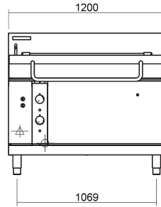
E580-12, E580-12E
