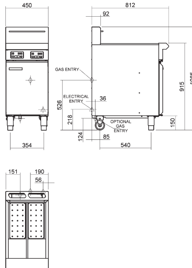
GT46E
